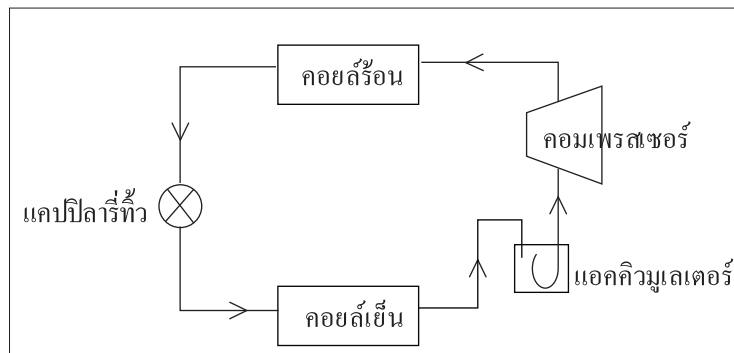
ผังวงจรวางน้ำยาของเครื่องปรับอากาศ
